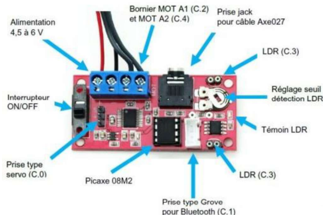
Figure 1 : carte Picaxe DGB (A4.fr)
